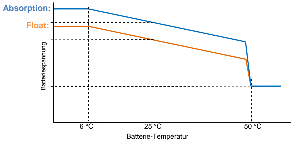
Abbildung 16 Grafik zum Temperatursgleich für die Spannungswerte der Ladeerhaltungs- und Konstant Spannungs-Phasen
