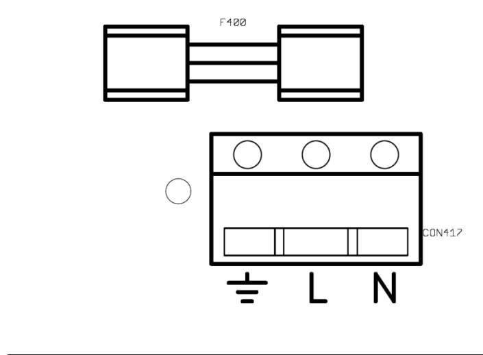
Afbeelding 6 Ingangsaansluiting voeding
