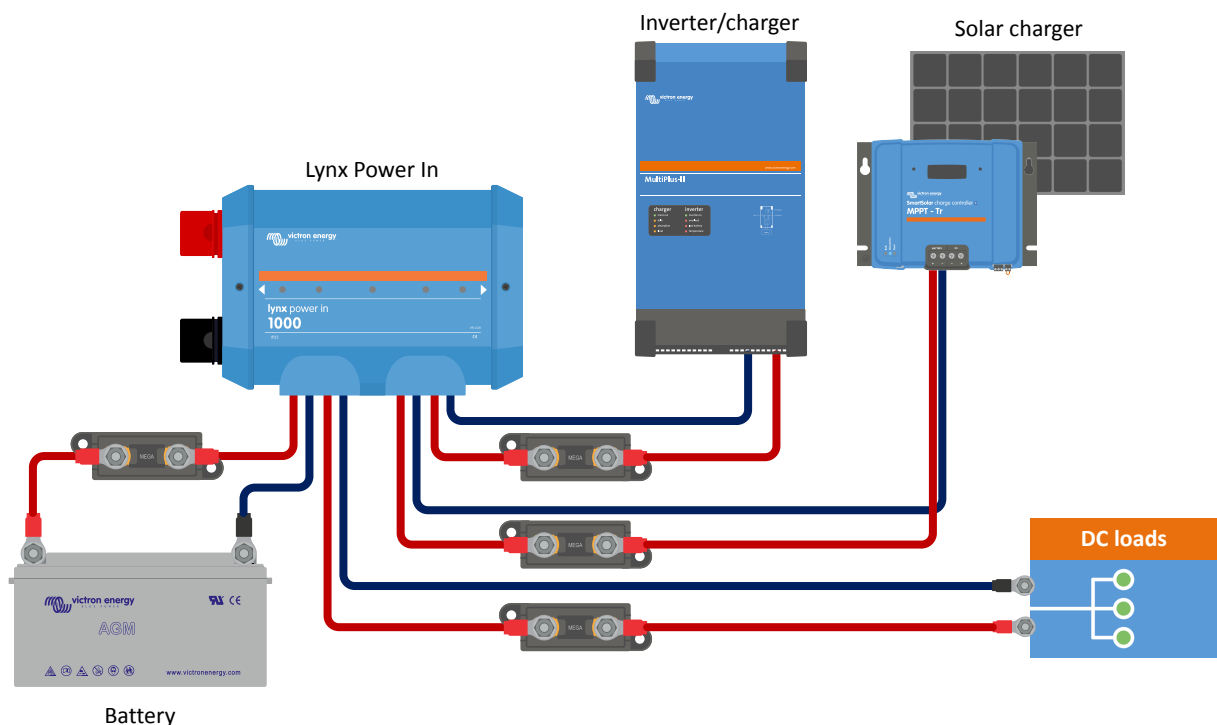
System met alleen een Lynx Power In
