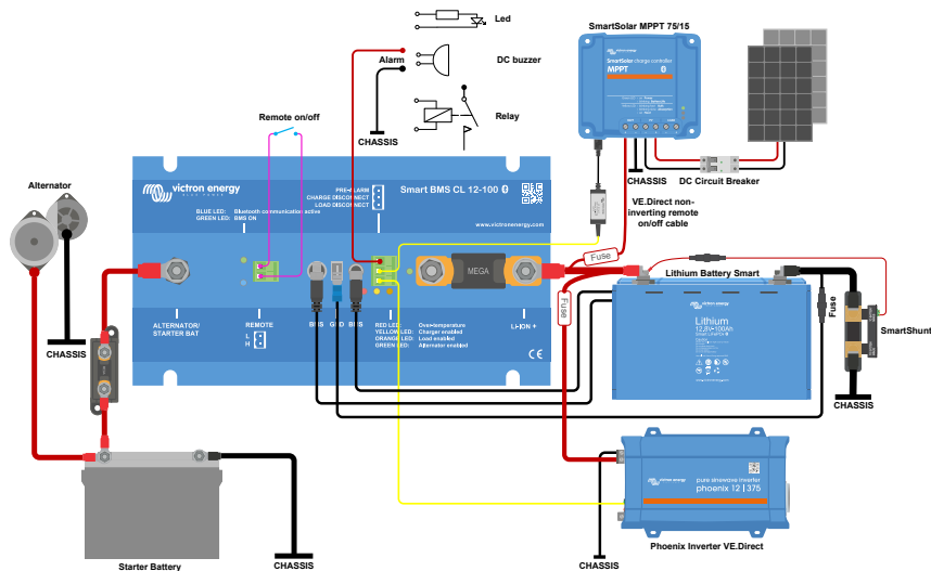
Afbeelding 2: Toepassingsvoorbeeld met een MPPT en een Phoenix omvormer
