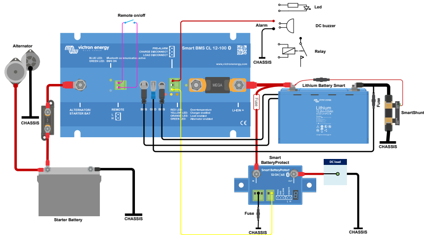
Afbeelding 1: Toepassingsvoorbeeld voor een voertuig of boot, met aan-/uitschakelaar tussen H en L
